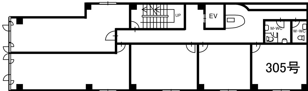
2~8階 平面図
